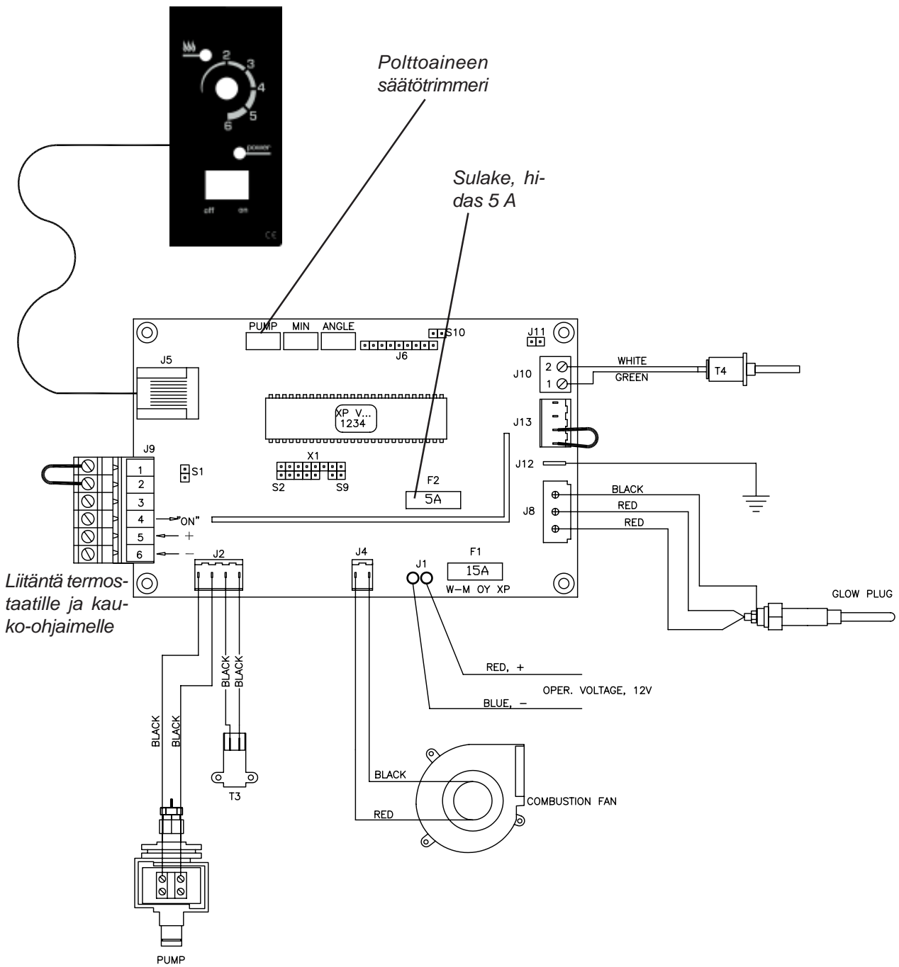
Kuva 17: Elektroniikkakortin liitännät.
