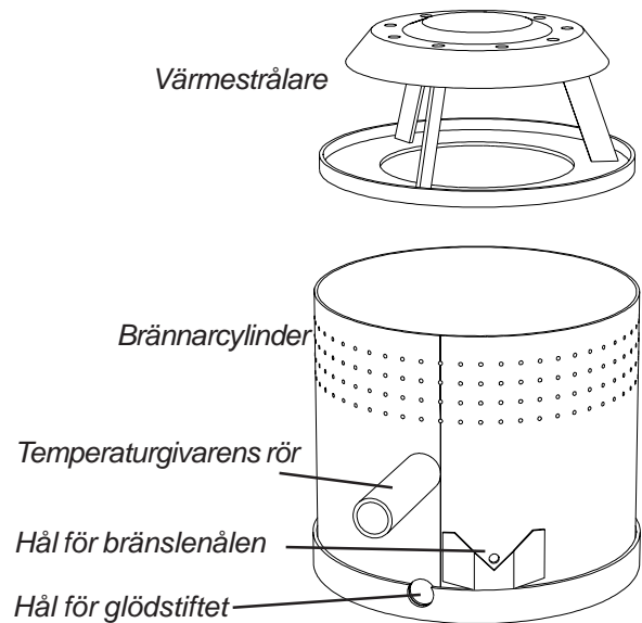
Figur 13: Demontering av värmestrålaren.
