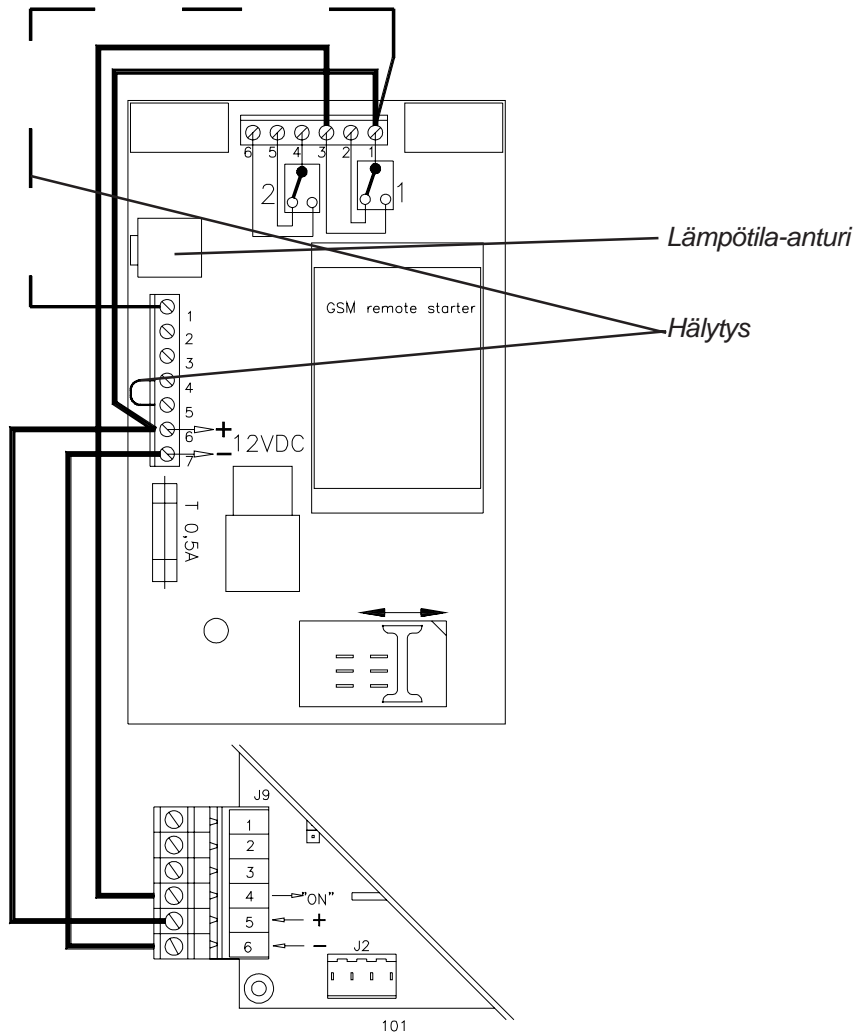
Kuva 19: Magneettiventtiilin kytkentä.
