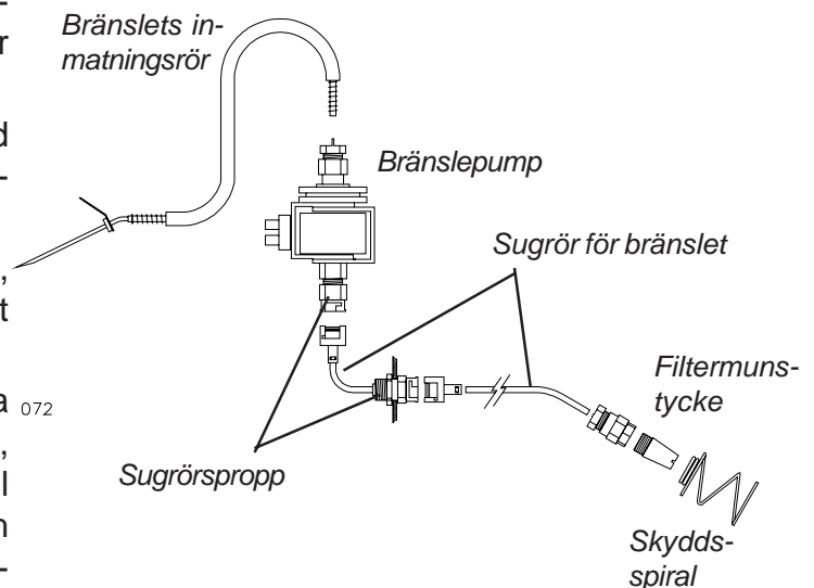
Figur 16: Bränslesystemets delar.
