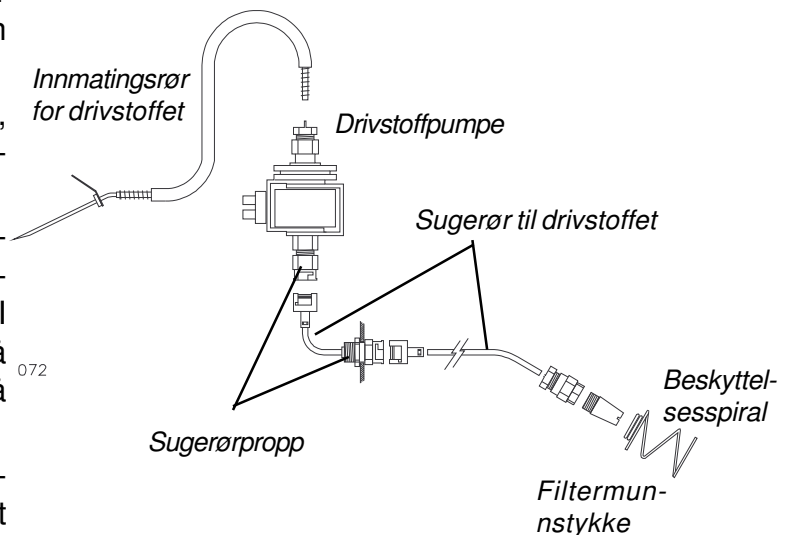
Bilde 16: Delene til drivstoffsystemet.
