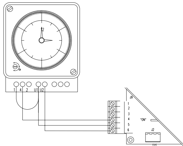
Figur 20. Anslutning av en rumstermostaten (a) och en mekanisk veckotimerneller (b).
