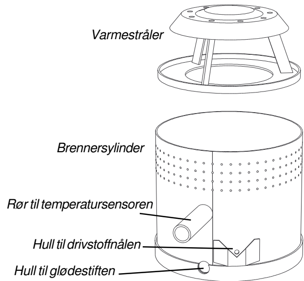
Bilde 12: Delene til brenneren M26.
