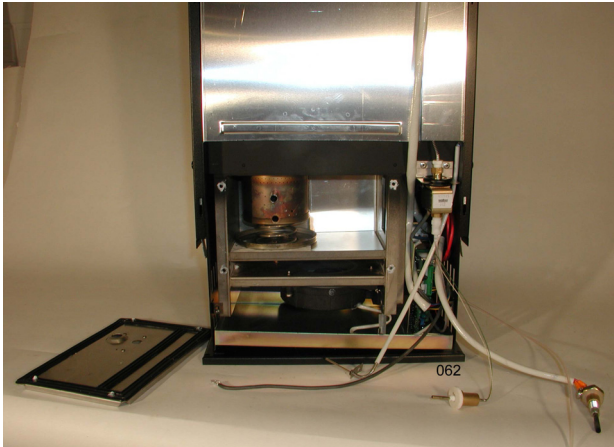
Figur 11: Brännarens lösgöring.
