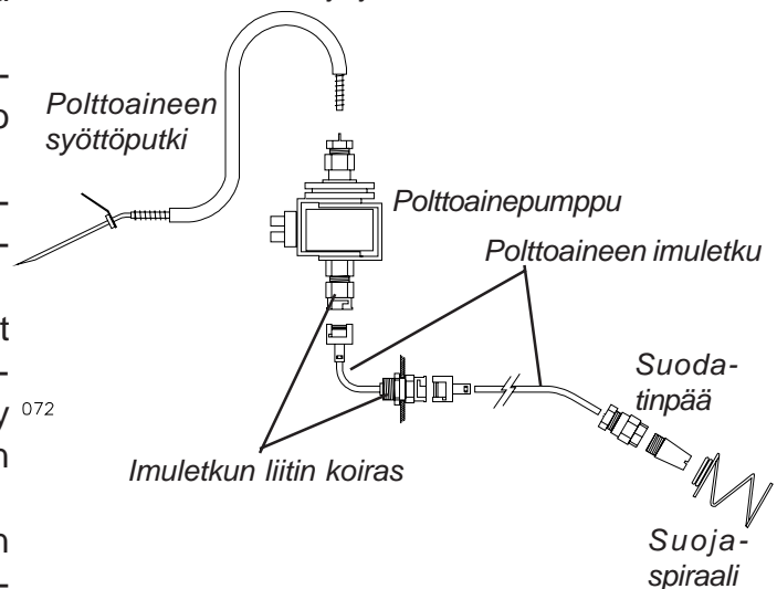
Kuva 16: Polttoainejärjestelmän osat.
